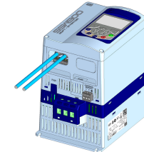
(i) Accessory connection (i) Conexión del accesorio (i) Conexão do acessório
