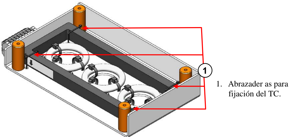
Figura 2: Instalación del TC de falta a tierra.
