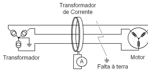
Figura 1 – Proteção de falta à terra por medição de corrente de fuga.
