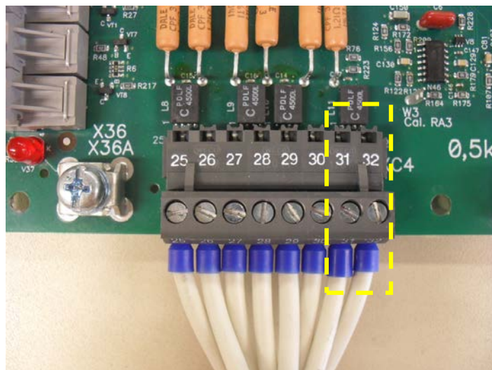
Figura 5 – Conexión del TC de falta a tierra a la tarjeta CSMx
