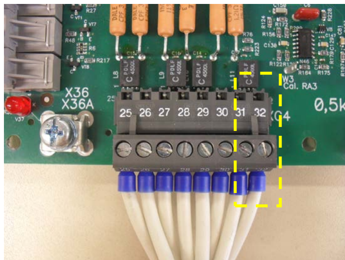
Figura 5 – Conexão do TC de falta à terra ao cartão CSMx
