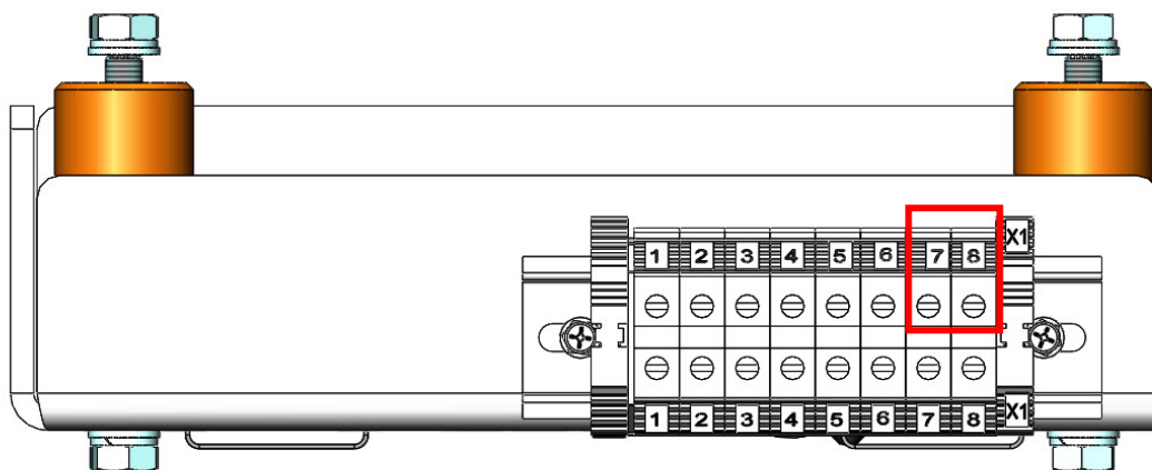
Figura 4: Terminais (7 e 8) para conexão dos cabos do TC de falta à terra.
