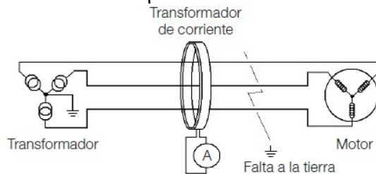
Figura 1 – Protección de falta a tierra por medición de corriente de fuga.
