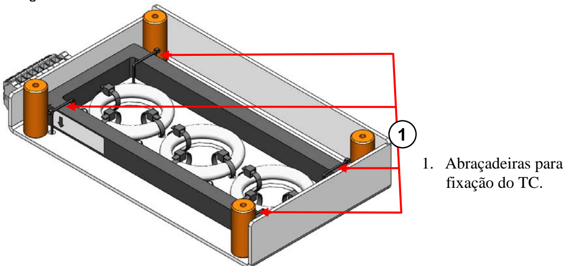
Figura 2: Instalação do TC de falta a terra.
