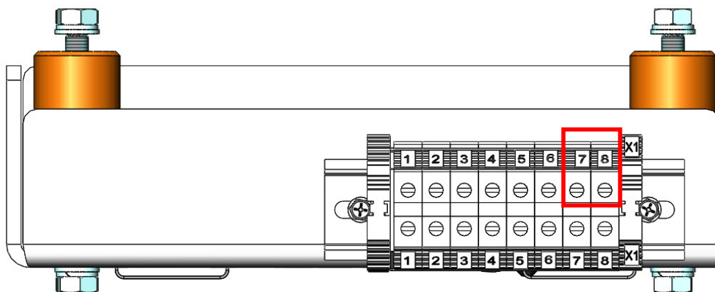
Figura 4: Terminales (7 y 8) para conexión de los cables del TC de falta a tierra.
