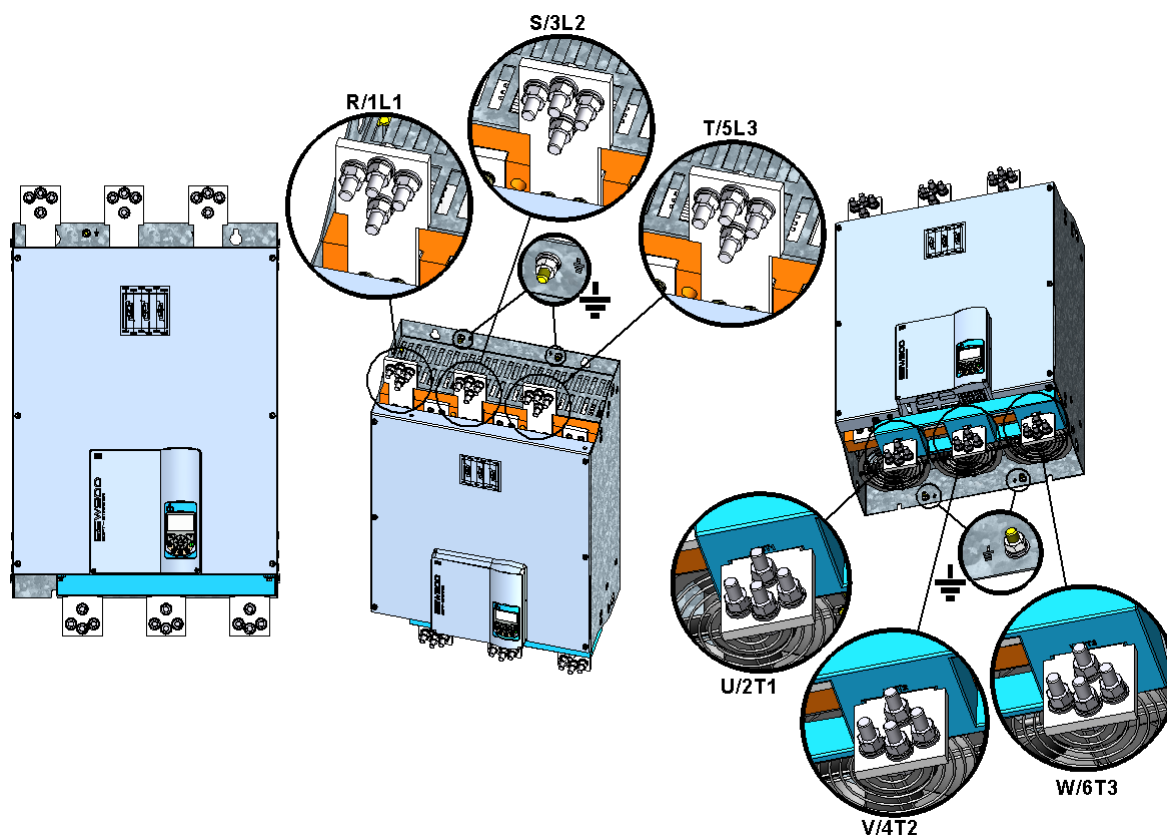
Figura 3.10: Bornes de potência e aterramento, mecânica G
