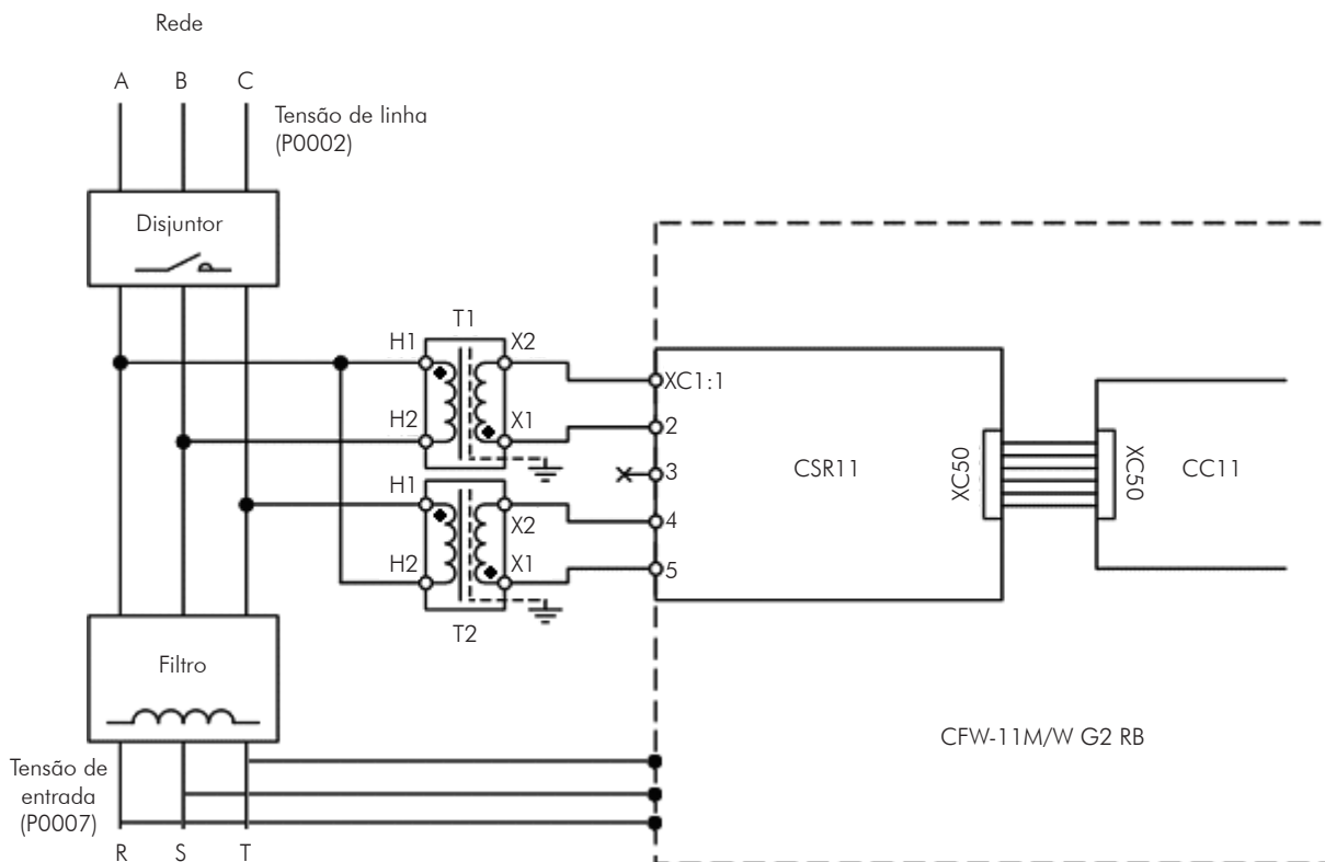
Figura 3.1 - Esquema de conexão do sincronismo
