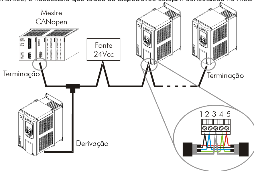
Figura 3.2: Exemplo de instalação em rede CANopen
