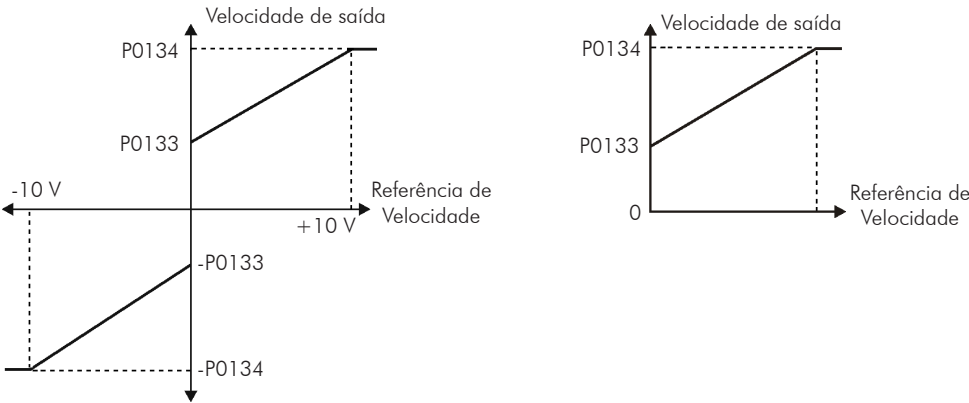
(a) Limites de velocidade considerando “Zona Morta” inativa (P0230 = 0)
