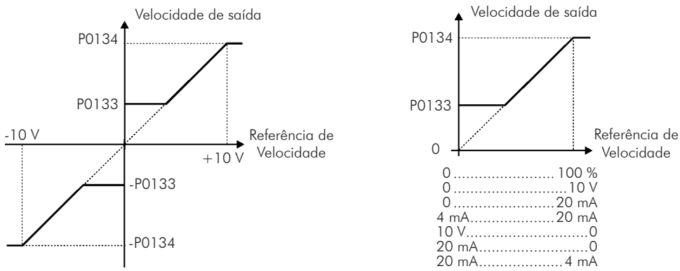
(b) Limites de velocidade considerando “Zona Morta” ativa (P0230 = 1)
