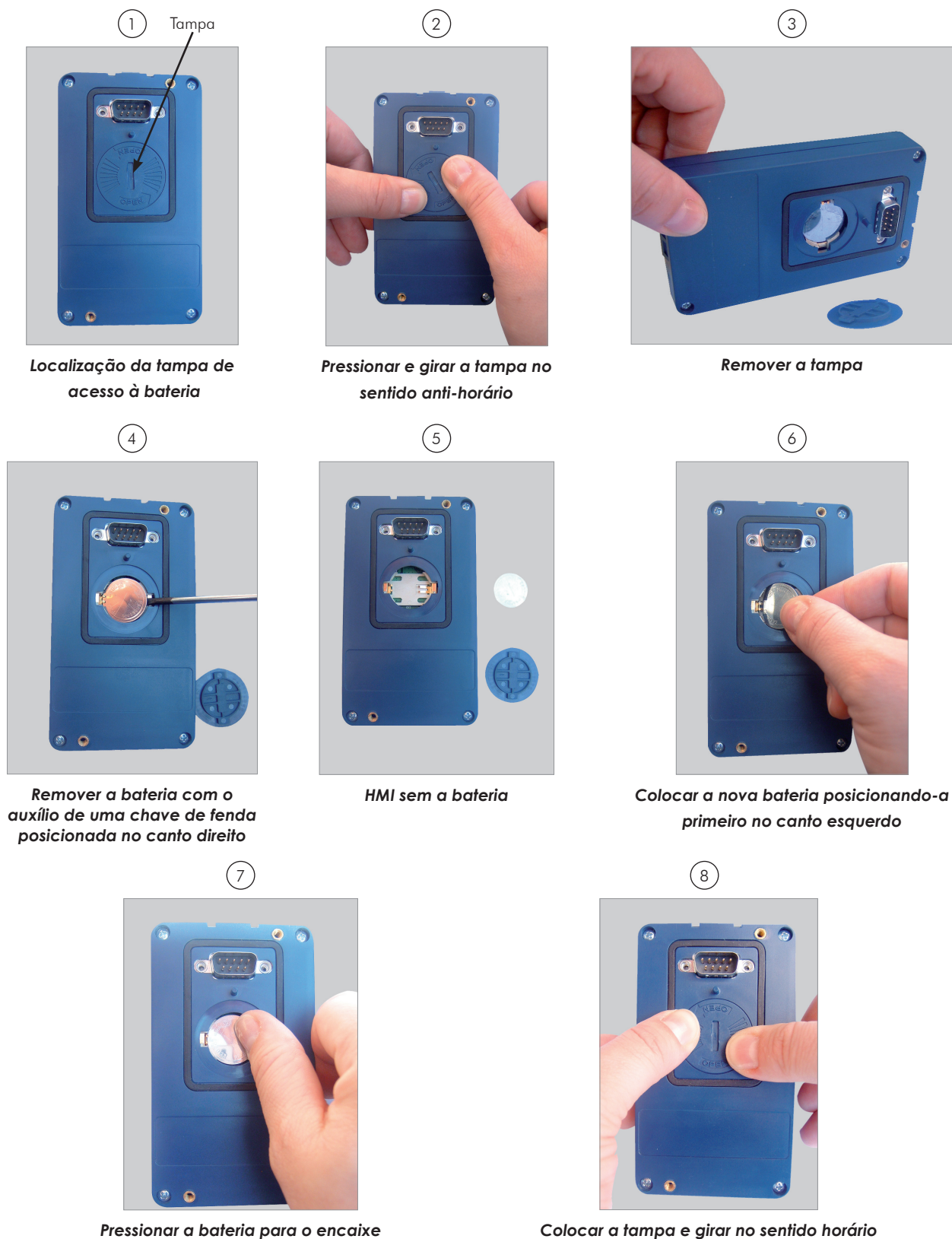
Figura 4.2 - Substituição da bateria da HMI
