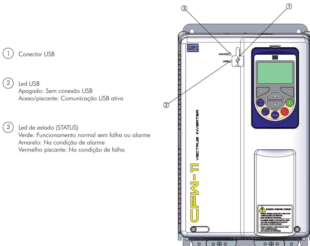
Figura 3.3 - LEDs e conector USB
