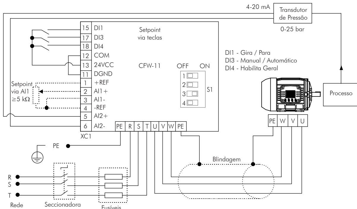
Figura 22.3 - Exemplo de aplicação do CFW-11 como regulador PID
