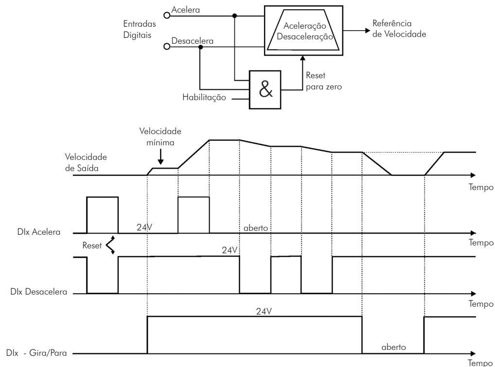
Figura 14.5 - Função do potenciômetro eletrônico (E.P.)
