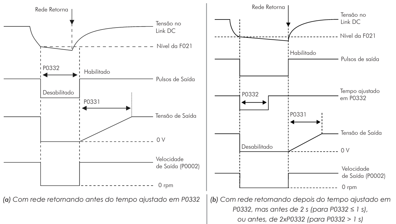
Figura 14.7 - (a) e (b) - Atuação do Ride-Through em modo V/f
