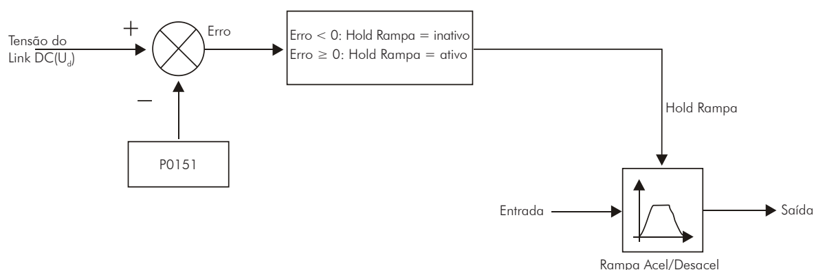
Figura 9.10 - Blocodiagrama da função de limitação da tensão do link DC utilizando Hold de Rampa
