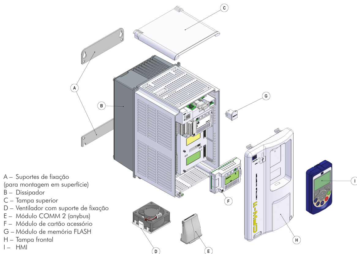
Figura 3.2 - Principais componentes do CFW-11
