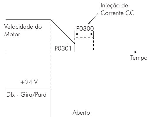
(b) Atuação da frenagem CC no bloqueio por rampa (via desabilita rampa)
