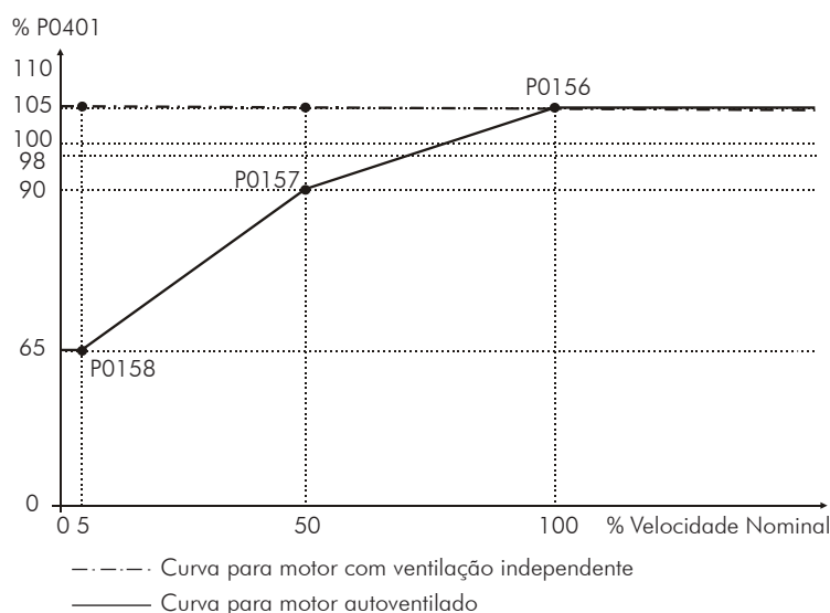
Figura 17.2 - Níveis de proteção de sobrecarga
