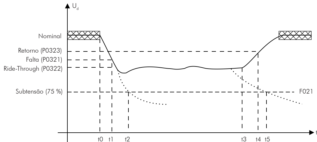
Figura 14.8 - Atuação da função Ride-Through em modo vetorial
