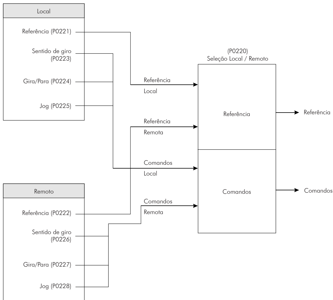
Figura 15.10 - Blocodograma Situação Local / Remoto
