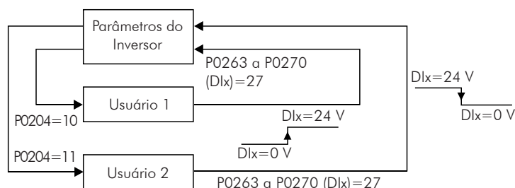
Figura 15.4 - Detalhes sobre o funcionamento da função Carrega Usuário 1/2
