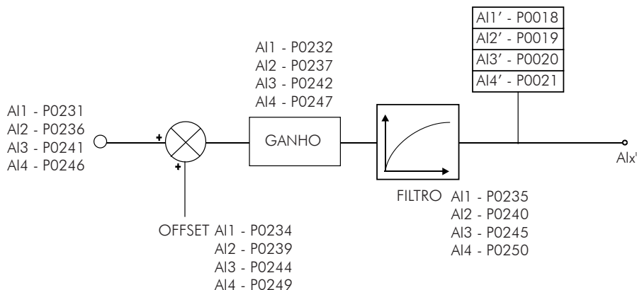
Figura 15.2 - Blocodiagrama das entradas analógicas
