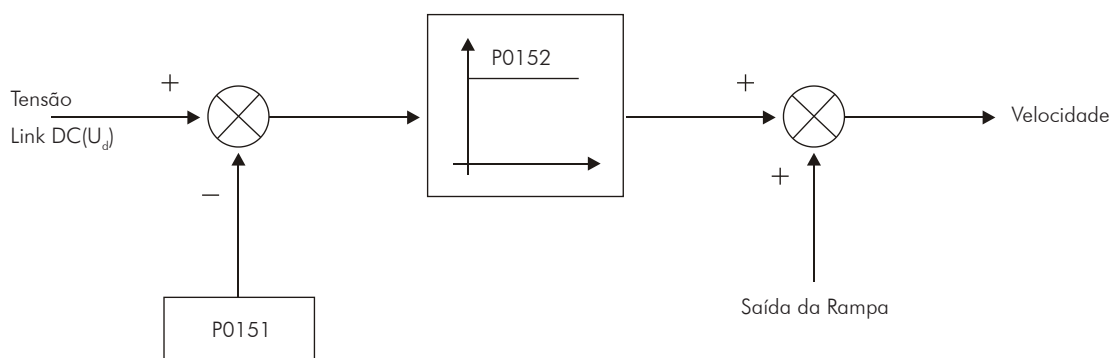
Figura 9.12 - Blocodiagrama da função de limitação da tensão do link DC via Acelera Rampa
