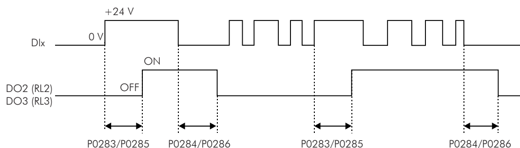
Figura 15.5 - Funcionamento da função temporizador DO2 (RL2) e DO3 (RL3)
