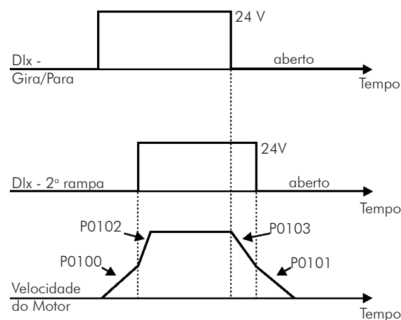
Figura 14.1 - Atuação da 2ª rampa
