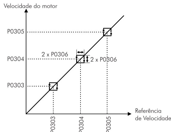
Figura 14.13 - Curva de atuação das “Velocidades Evitadas”
