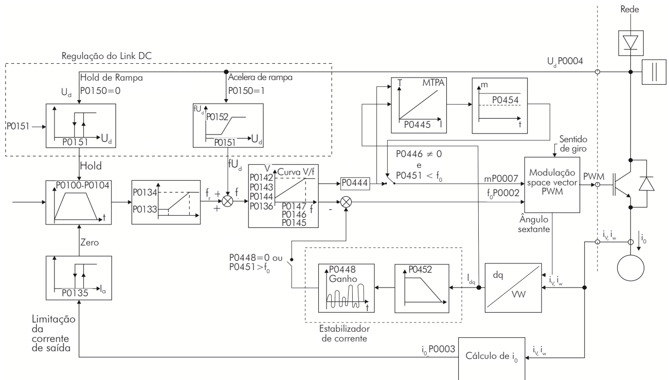
Figura 13.1 - Diagrama de blocos do controle VW PM
