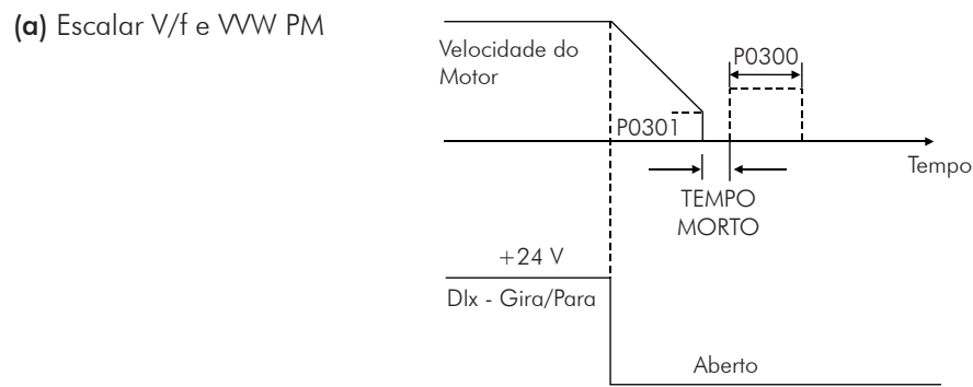
(a) Atuação da frenagem CC no bloqueio por rampa (via desabilita rampa)
