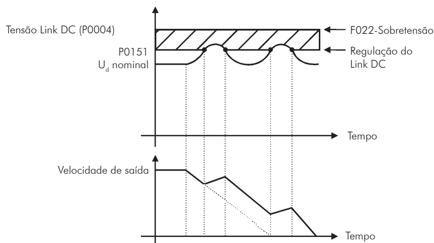
Figura 9.13 - Gráfico exemplo de atuação da limitação da tensão do link DC com a função Acelera Rampa
