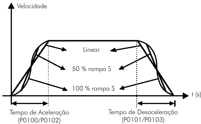
Figura 14.2 - Rampa S ou linear
