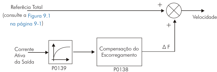
Figura 9.5 - Blocodiagrama da compensação de escorregamento
