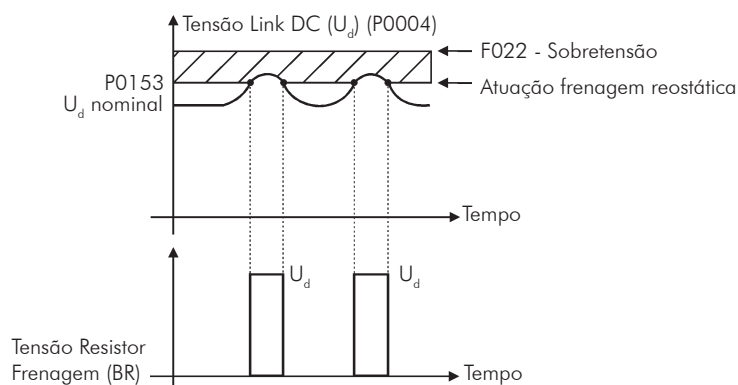
Figura 16.1 - Curva de atuação da Frenagem Reostática
