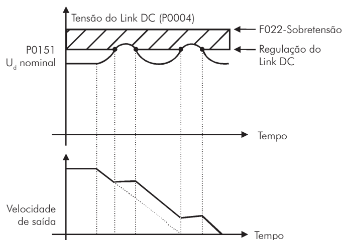
Figura 9.11 - Gráfico exemplo de atuação da limitação da tensão do link DC com a função Hold de Rampa
