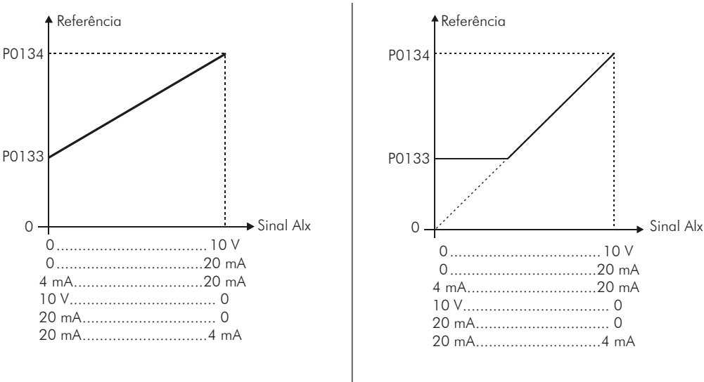
(a) Atuação das Entradas Analógicas com Zona Morta Inativa (b) Atuação das Entradas Analógicas com Zona Morta Ativa
