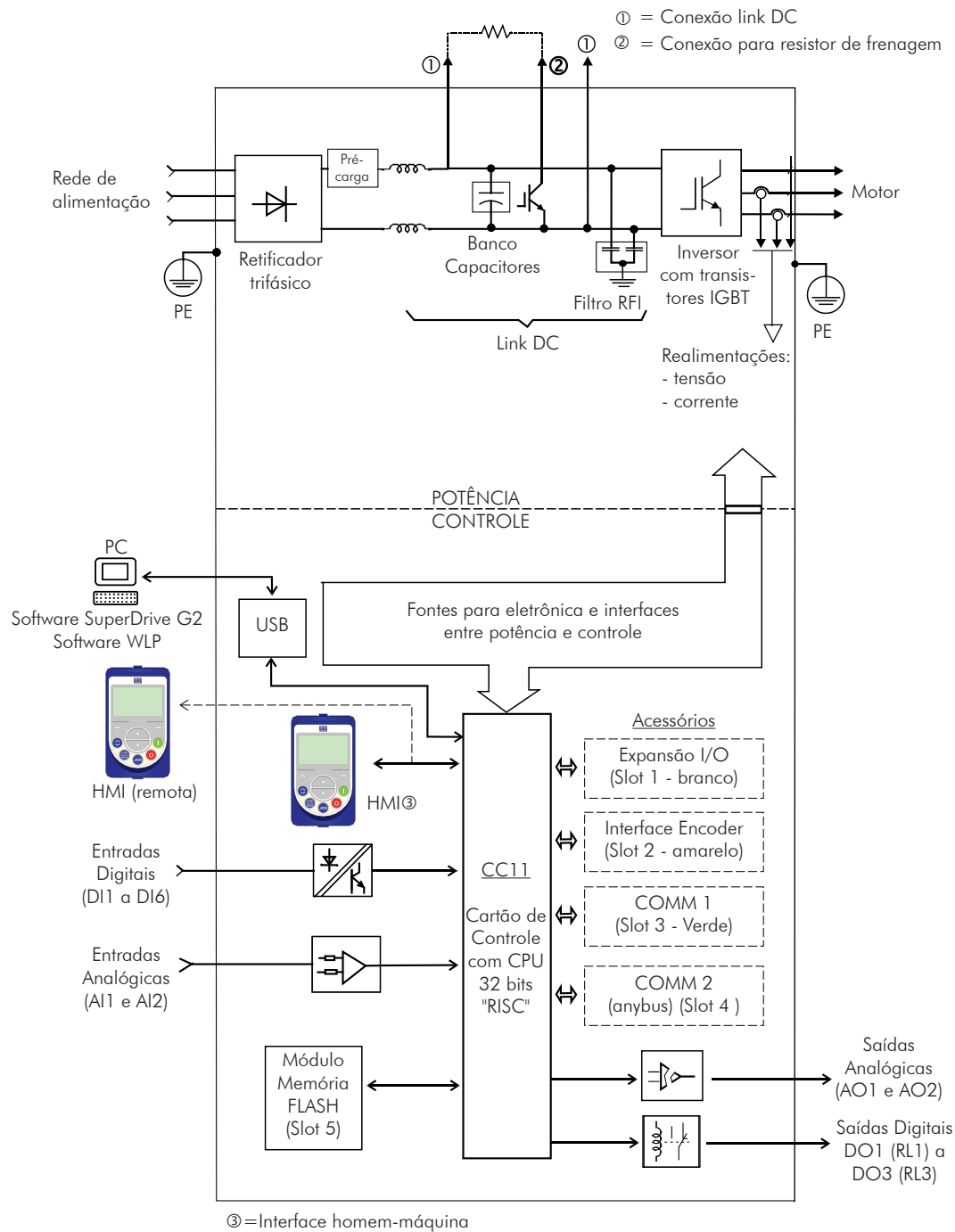
Figura 3.1 - Blocodiagrama do CFW-11
