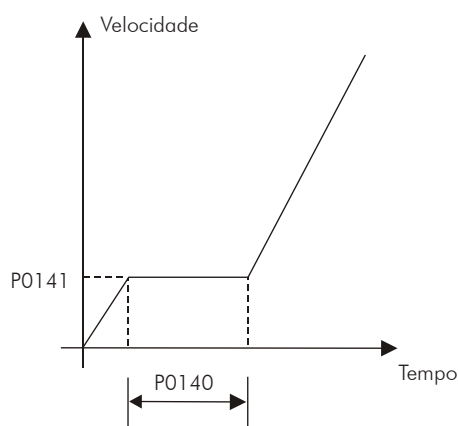
Figura 9.7 - Perfil da velocidade na aceleração em função de P0140 e P0141
