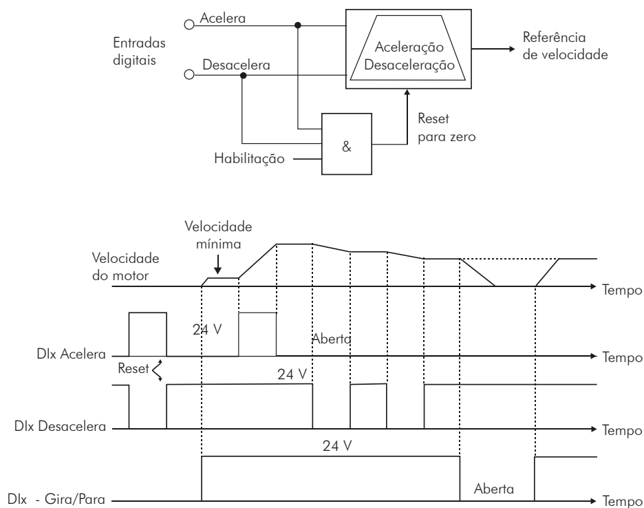
Figura 15.6 - (a) a (m) - Detalhes sobre funcionamento das funções das Entradas digitais
