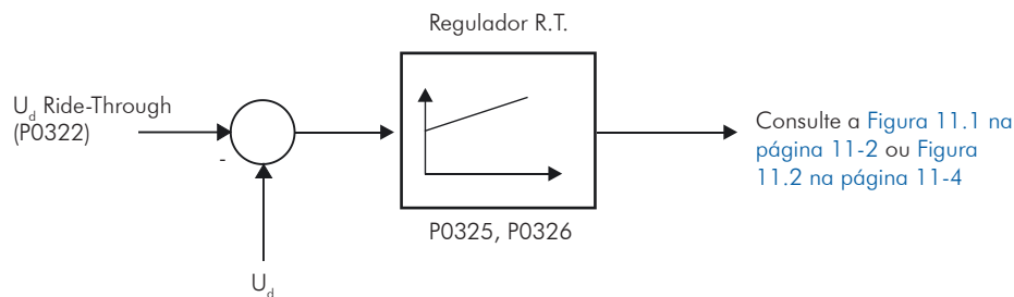
Figura 14.9 - Controlador PI do Ride-Through
