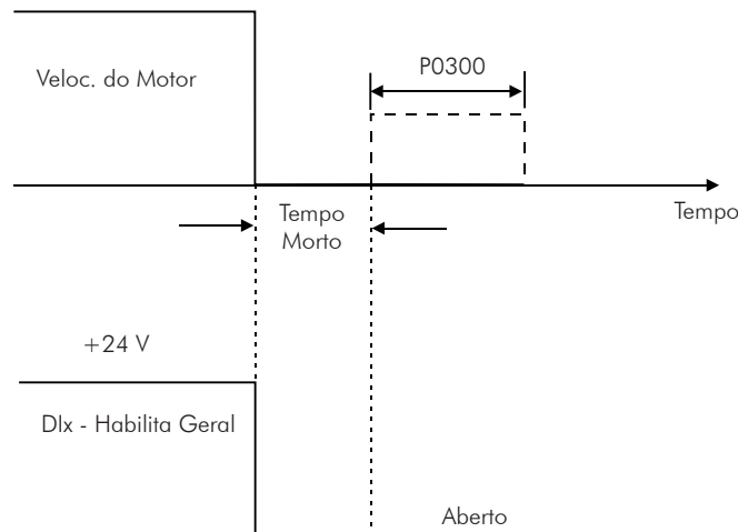
Figura 14.12 - Atuação da frenagem CC via Desabilita Geral - Modo V/f
