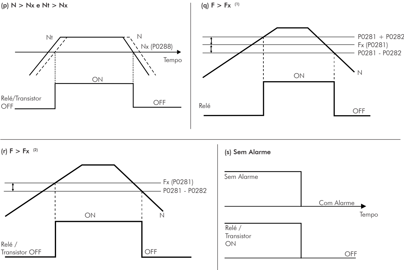
Figura 15.8 - (a) a (s) - Detalhes do funcionamento das funções das saídas digitais e a relé
