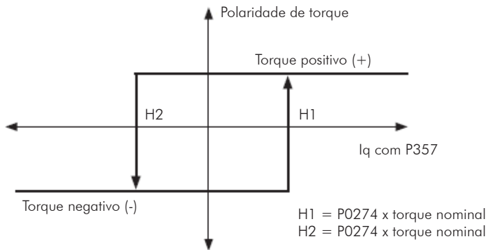
Figura 15.7 - Histerese para Corrente de Torque - Iq
