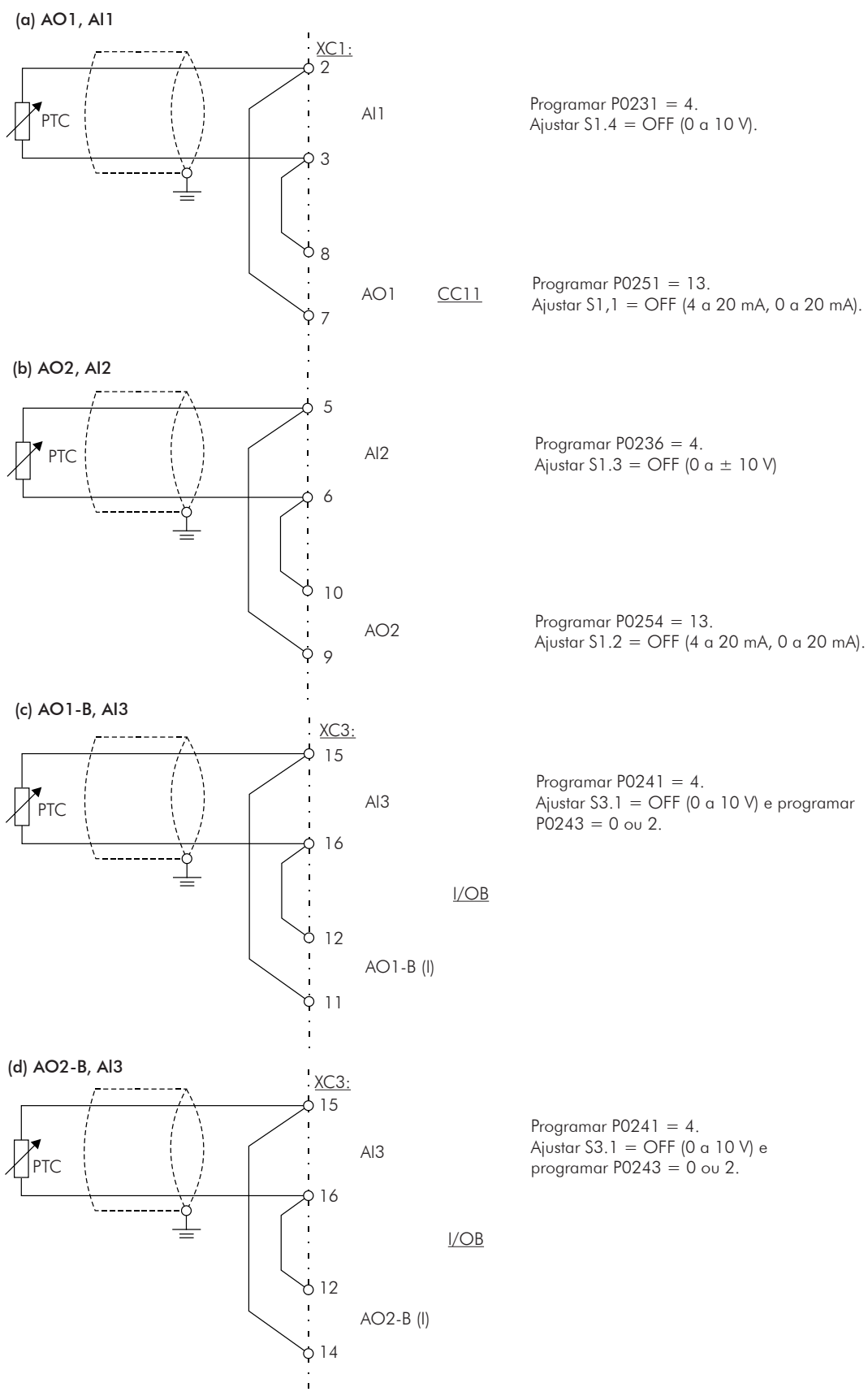
Figura 17.1 - (a) a (d) - Exemplos de conexões do PTC
