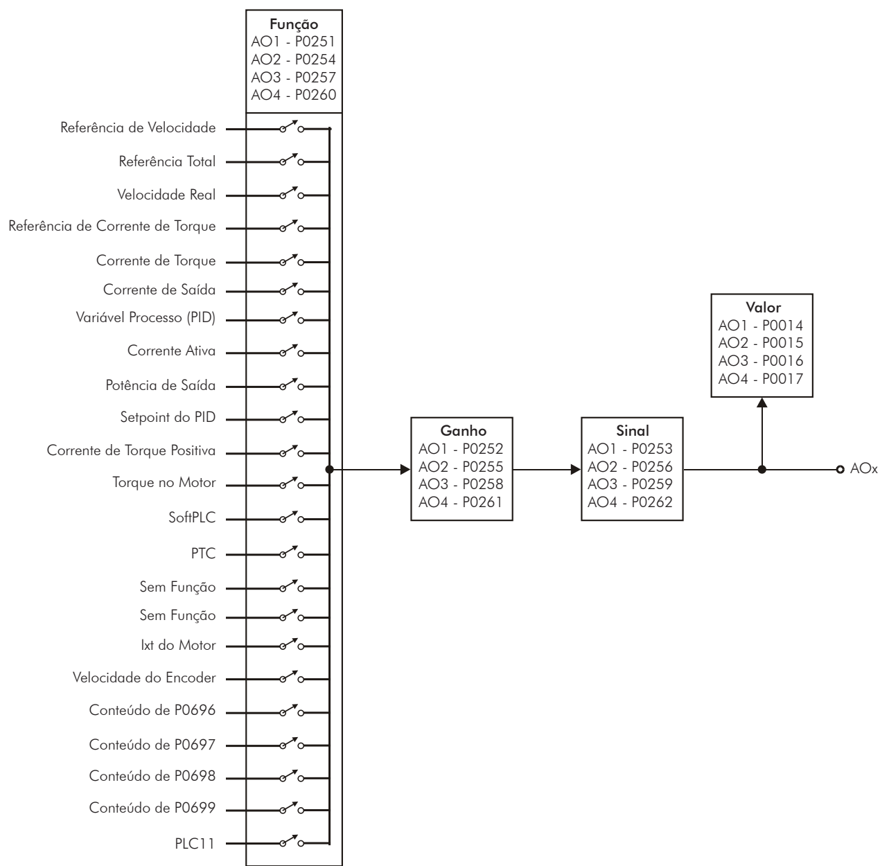
Figura 15.3 - Blocodiagrama das saídas analógicas
