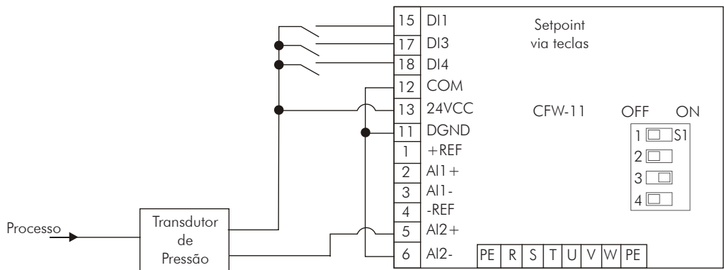
Figura 22.5 - Ligação de transdutor ao CFW-11 com 2 fios
