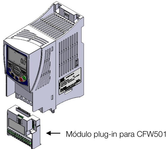
Figura 2.1: Ejemplo de accesorio de interfaz para CFW501
